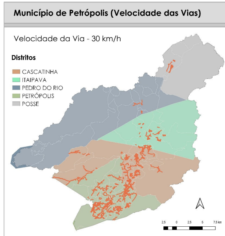
Figura 3.11: Vias Locais (Velocidade - 30 km/h)
